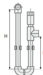
Расчёт высоты сифона (рис. 12)
